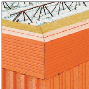
Rationelles Verlegen der Deckenrand-Systeme in einem Arbeitsschritt. Kein Zeitverlust durch Einschalungsarbeiten.
