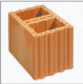
Der PFZ macht Anfänger überflüssig - ein Schnitt durch die Lochreihe im Mittelsteg schafft exakt 2 halbe Ziegel. Ecken, Türlaibungen und Aufzugsschächte können so noch leichter hergestellt werden als bisher.
